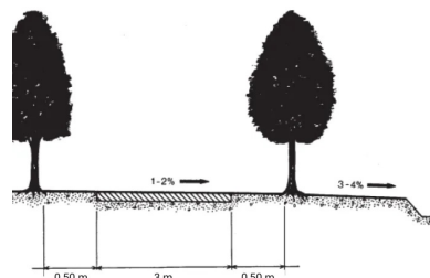
Profil en travers de la voie verte entre Jonquières et Orange.
