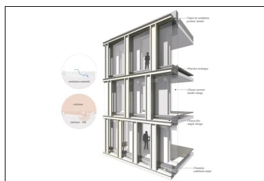
Façade double peau, clapet de ventilation en position fermée
