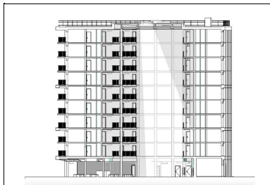
4. Coupe transversale sur l'atrium
